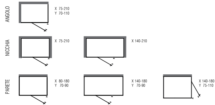
h. 195 cm vetro temperato trasparente 8 mm tempered transparent glass / cristal templado transparente
