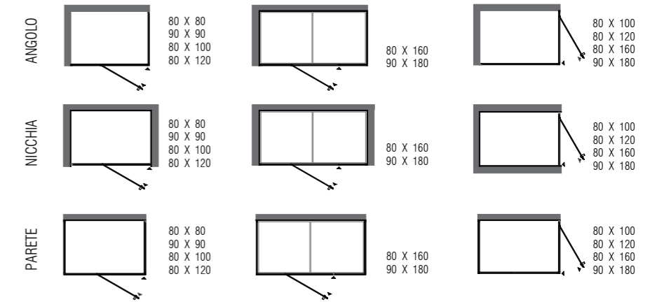
h. 200 cm vetro trasparente temperato extrachiaro 10 mm tempered transparent extraclear glass / cristal transp. templado extraclaro
