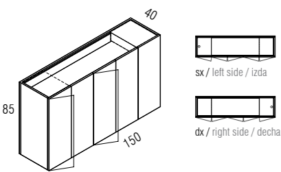
150_5 ante / doors / puertas
