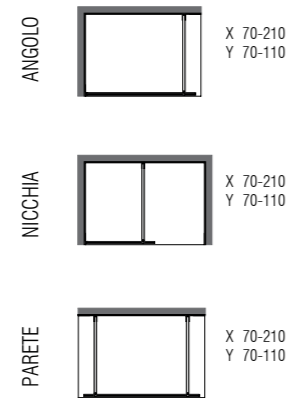
h. 195 cm vetro temperato trasparente 8 mm tempered transparent glass / cristal templado transparente
