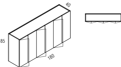
180_6 ante / doors / puertas
