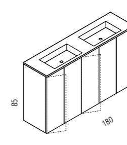
doppio / double / doble
