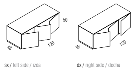
120_3 ante / doors / puertas
