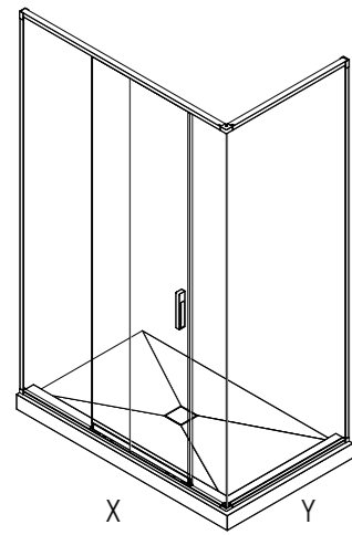
LAMA - box doccia vetro fisso shower screen / cristal fijo
