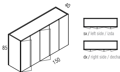
150_5 ante / doors / puertas
