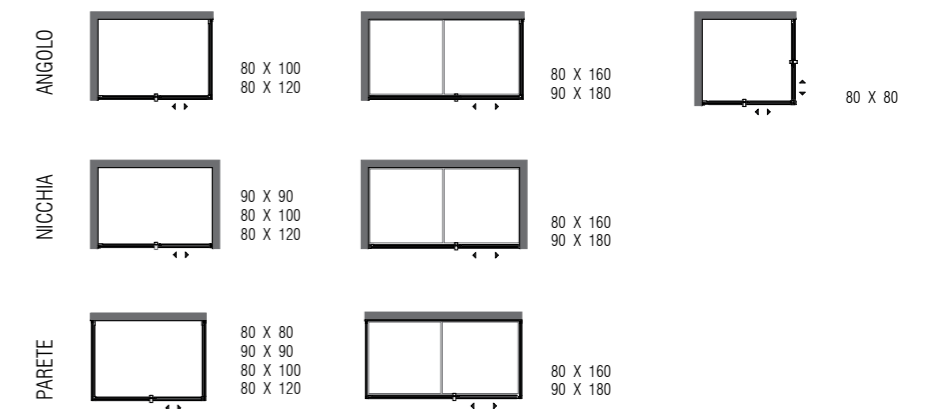
h. 200 cm vetro trasparente temperato extrachiaro 10 mm tempered transparent extraclear glass / cristal transp. templado extraclaro
