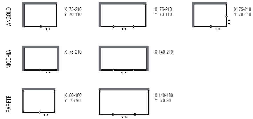
h. 195 cm vetro temperato trasparente 8 mm tempered transparent glass / cristal templado transparente
