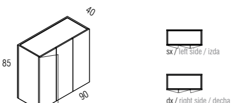
90_3 ante / doors / puertas
