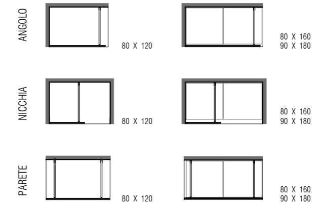
h. 200 cm vetro trasparente temperato extrachiaro 10 mm tempered transparent extraclear glass / cristal transp. templado extraclaro
