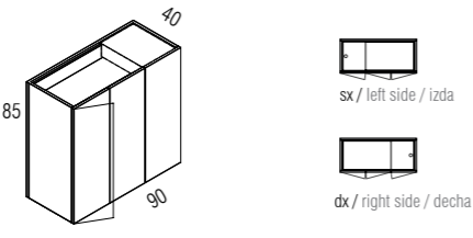
90_3 ante / doors / puertas
