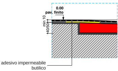
particolare_A
