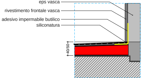
particolare_B
