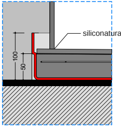
particolare_B
