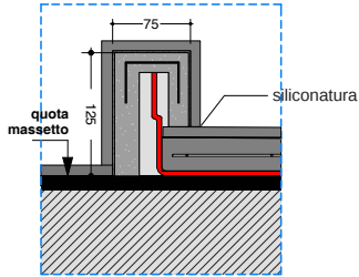
particolare_A
